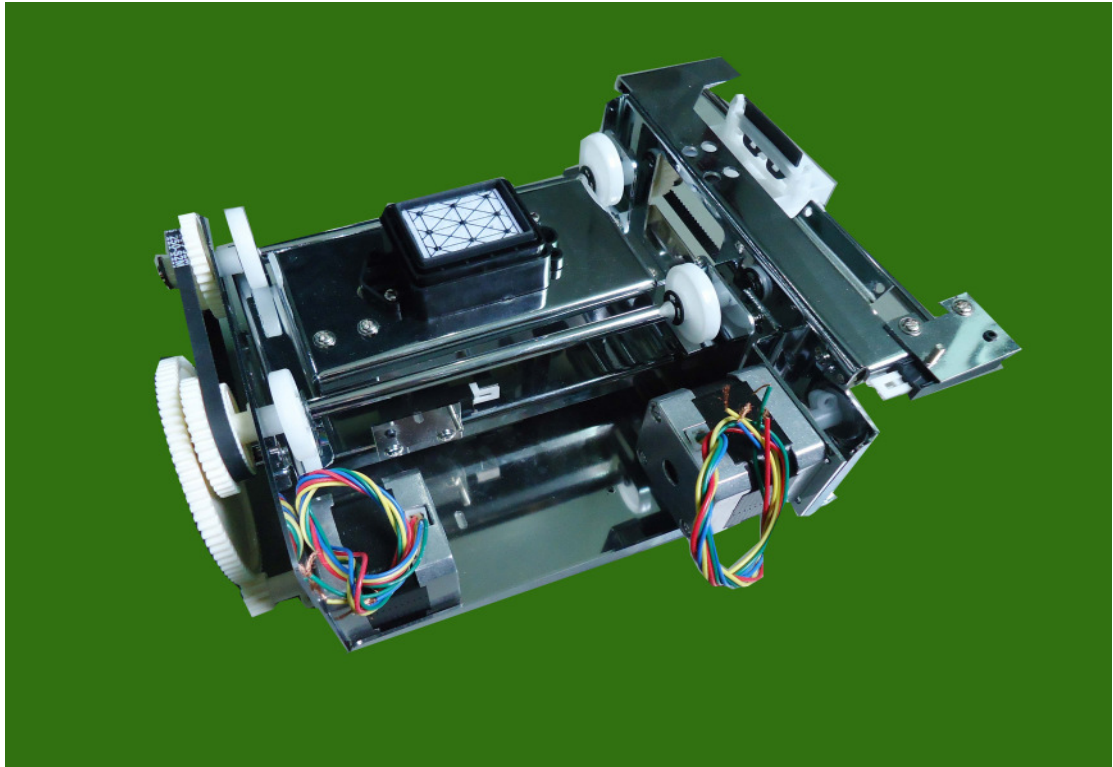
单头升降式墨栈
