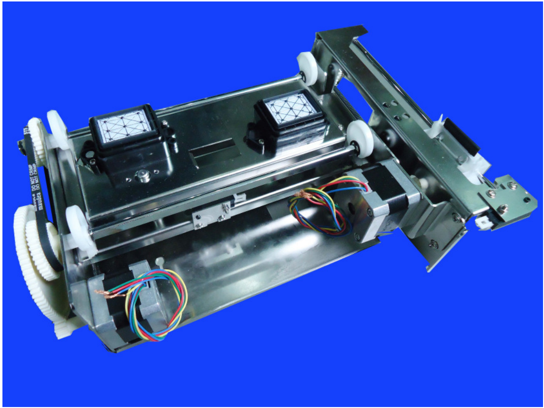
双头单升墨栈
