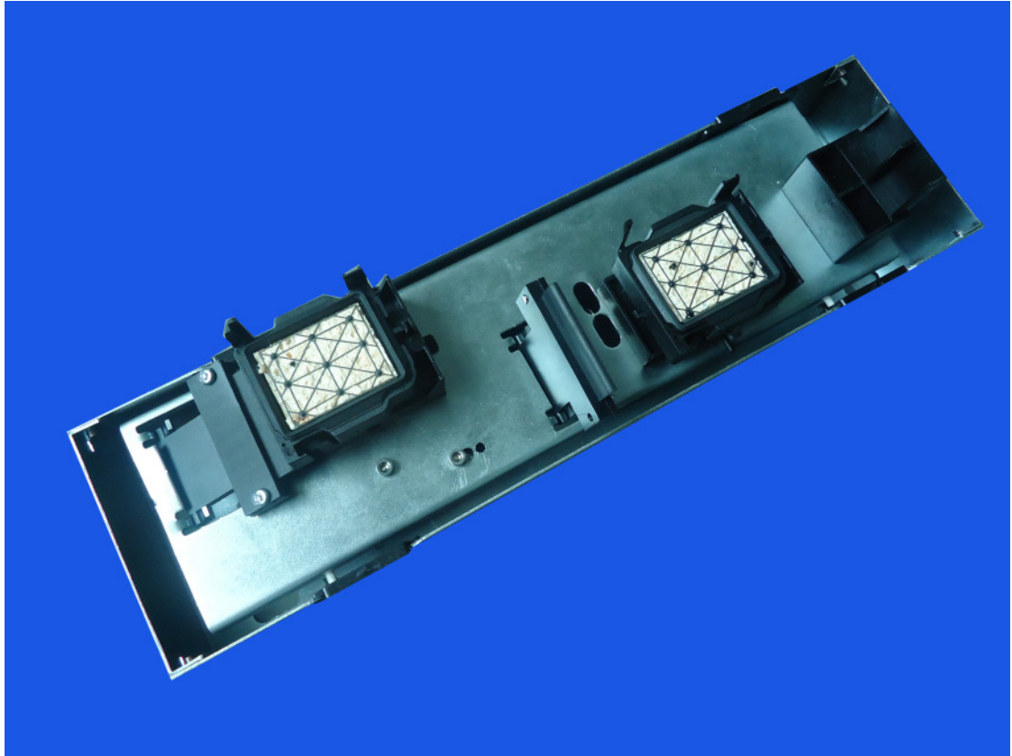
五代头双头墨栈
